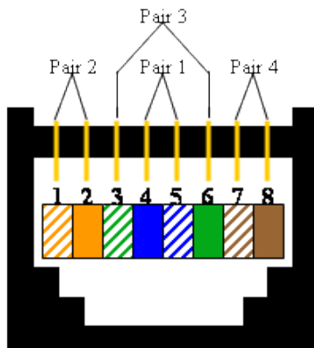
T568B
